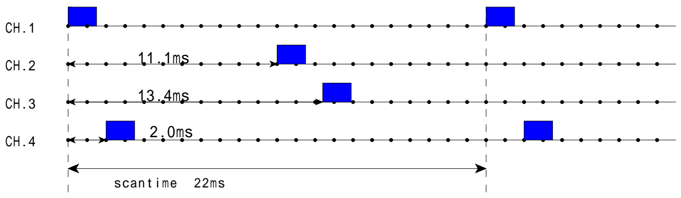
2.4GHz 4ch.Reciebar output Timechart (J)
