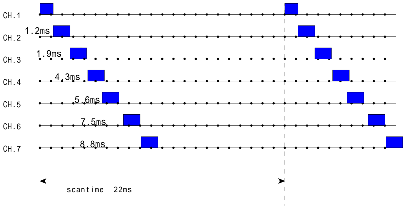
2.4GHz Telemetry sys. 7ch.Reciebar output Timechart (H)
